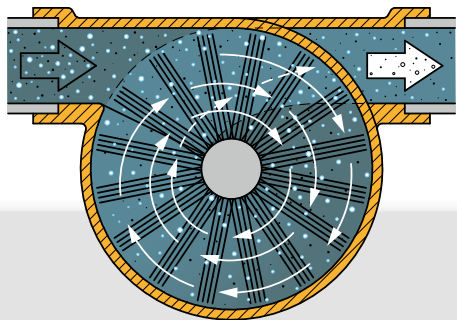
Konvencionalni ločevalnik s celotnim pretokom: ločevanje največ 25% na cikel.
